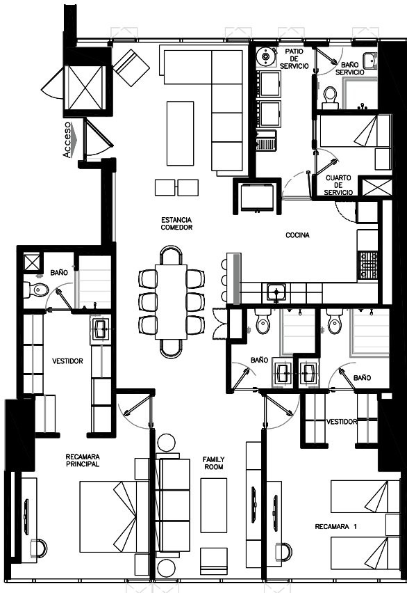
Planta arquitectonica-Amueblado
