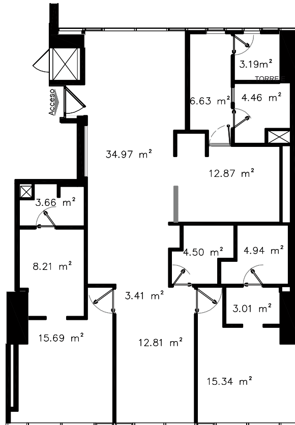
Planta arquitectonica-Distribución
